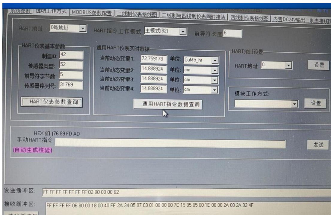
4.SM100-B 配置软件读到的 HART 仪表实时数据
